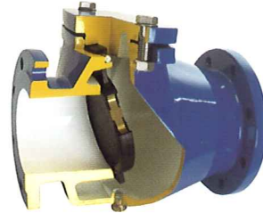
Scharnierende terugslagklep
